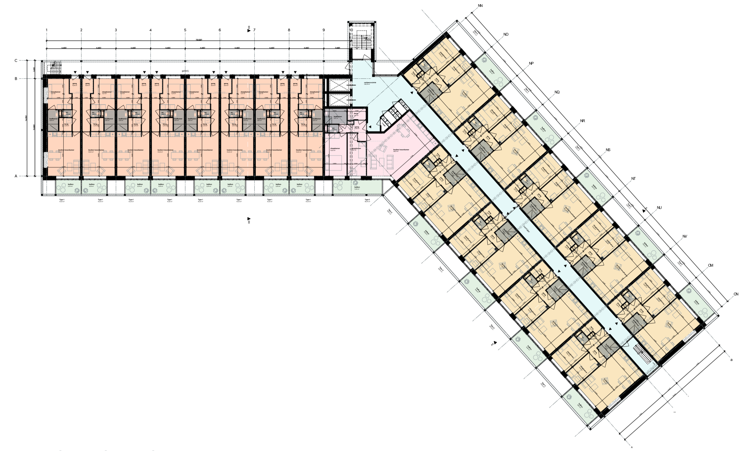
standaard verdieping
