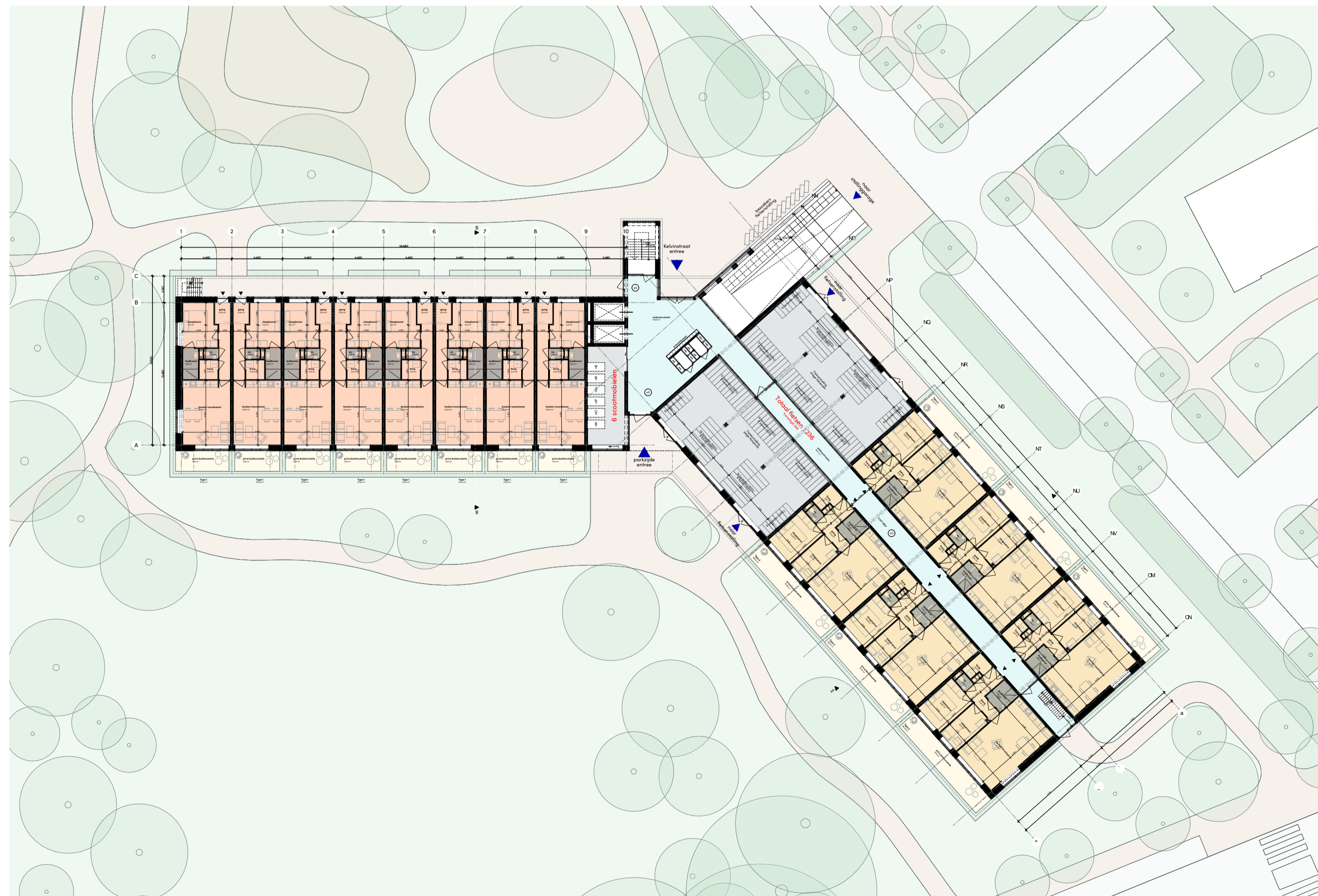
begane grond
