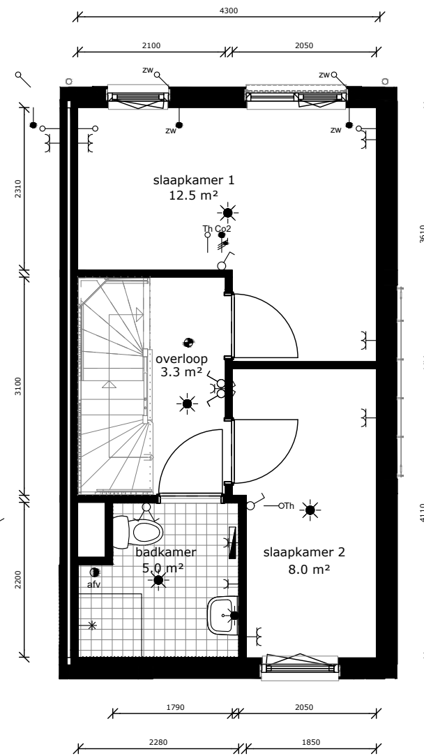
1e verdieping
