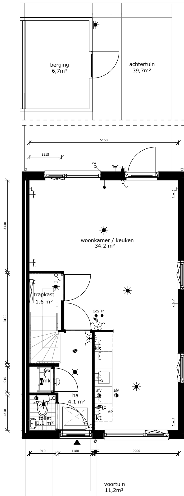
begane grond
