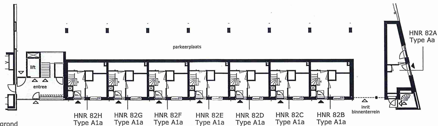
begane grond
