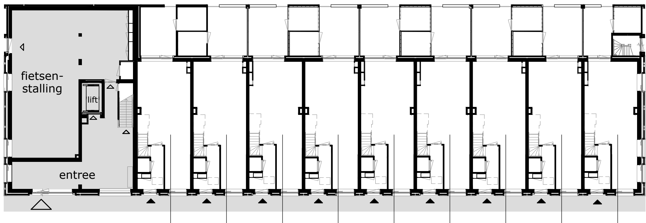
begane grond
