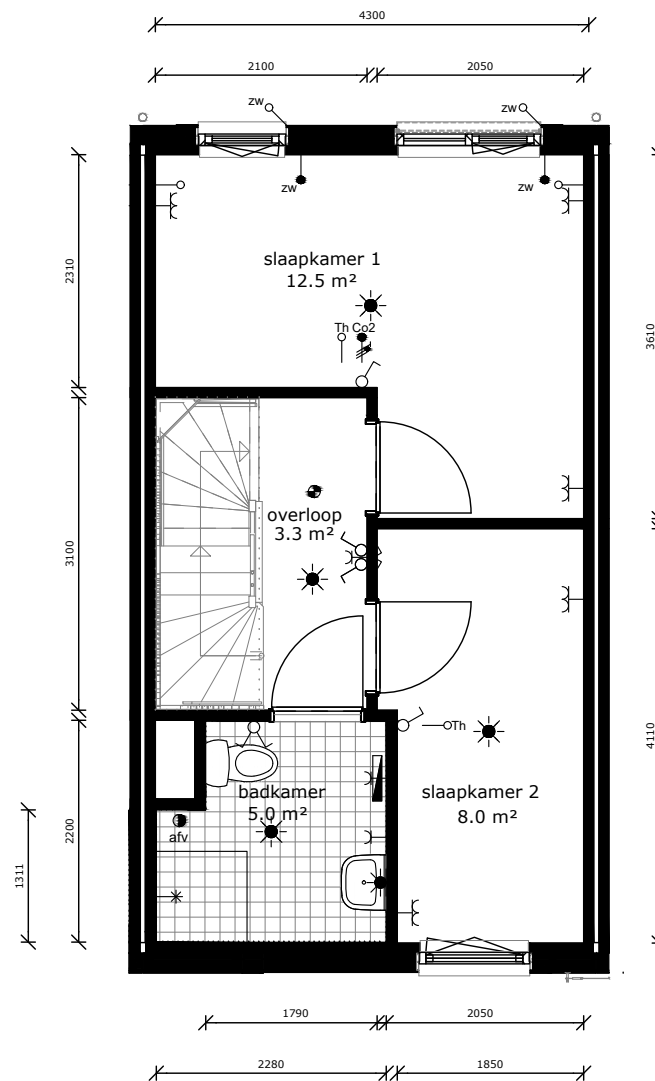
1e verdieping
