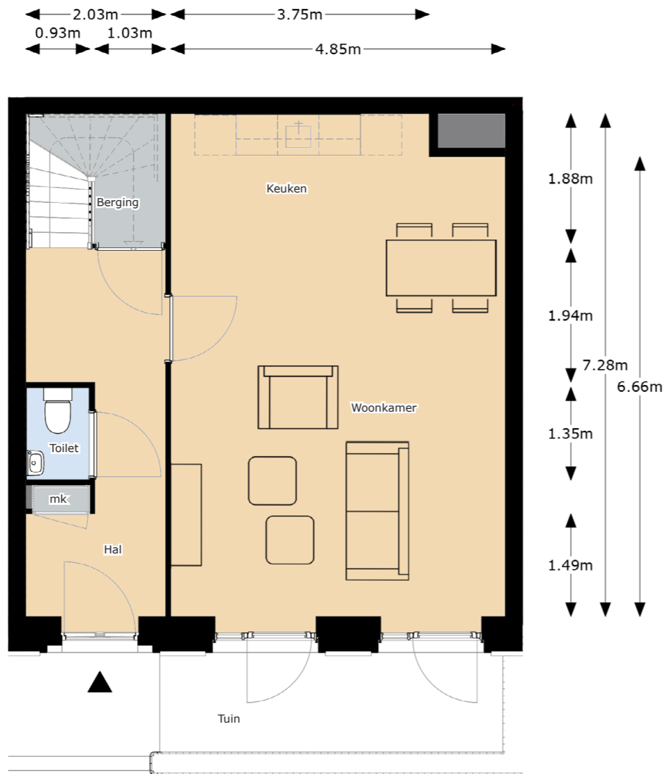
begane grond
