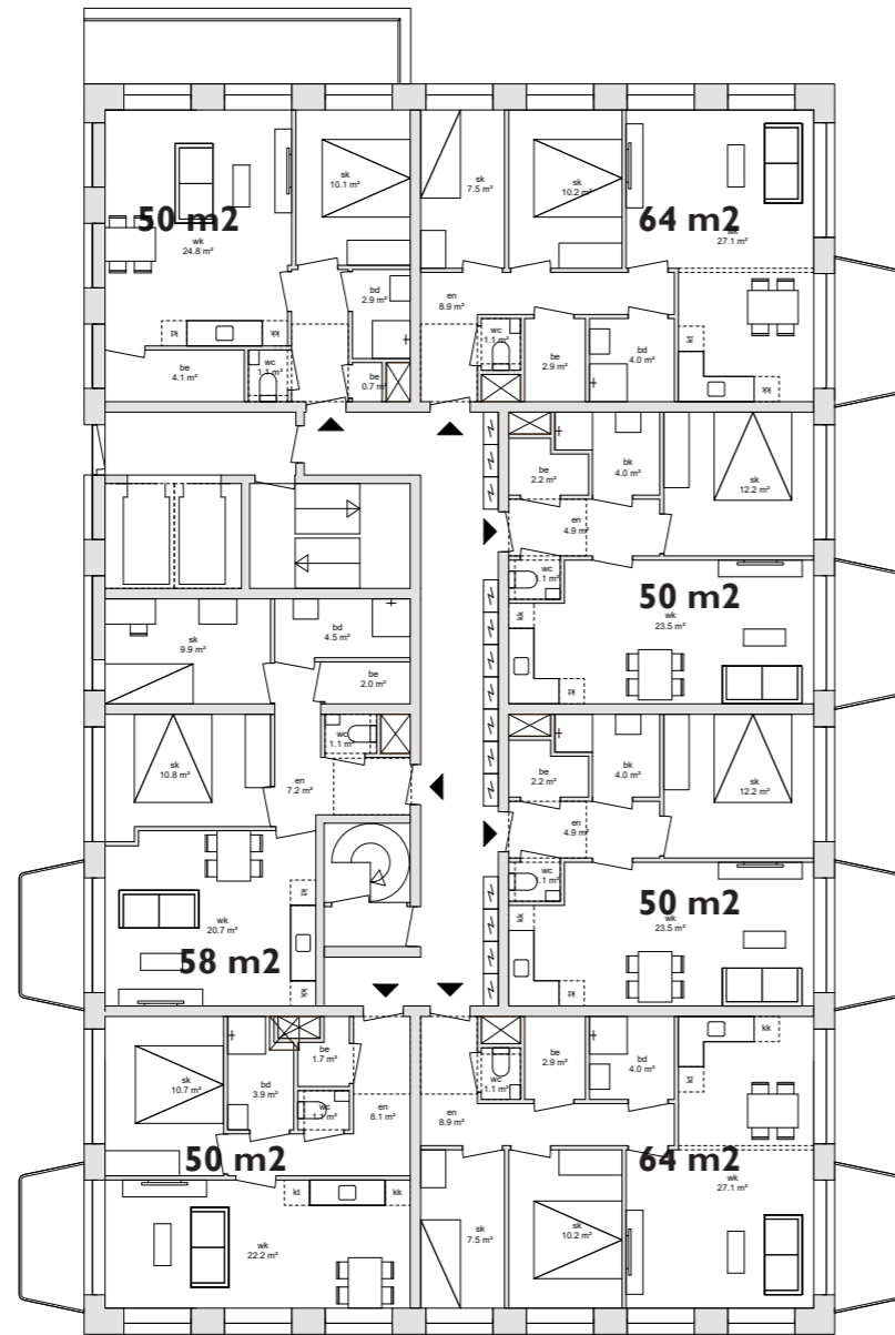
2E/M 4EVERDIEPING
