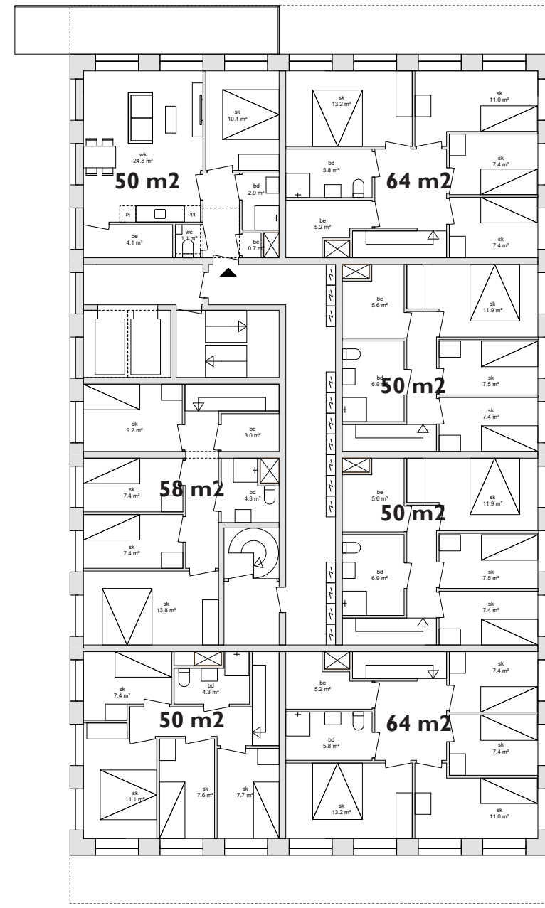
1E VERDIEPING
