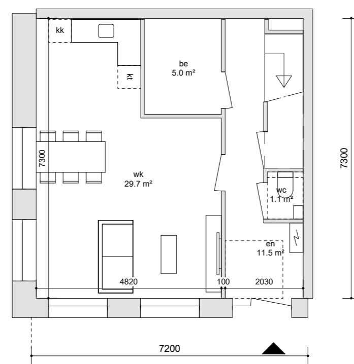
BEGANE GROND
