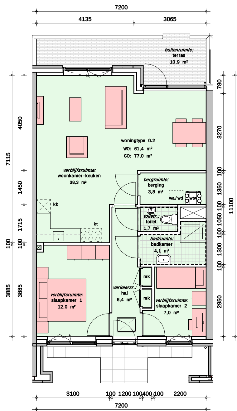
type 0.2 vrije hoogte 3260mm
