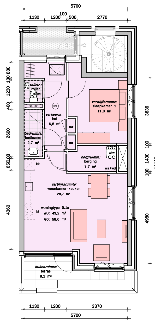
type 0.1a vrije hoogte 3260mm
