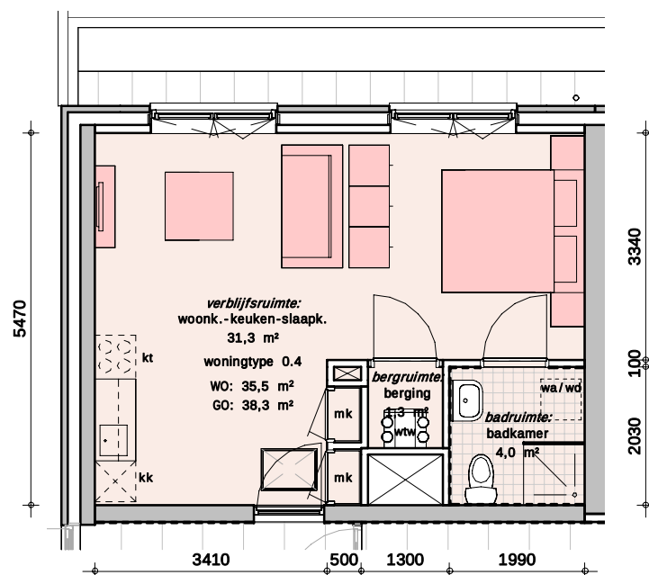
type 0.4 vrije hoogte 3260mm
