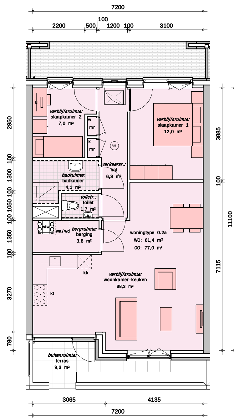
type 0.2a vrije hoogte 3260mm
