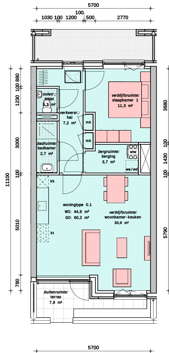
type 0.1 vrije hoogte 3260mm
