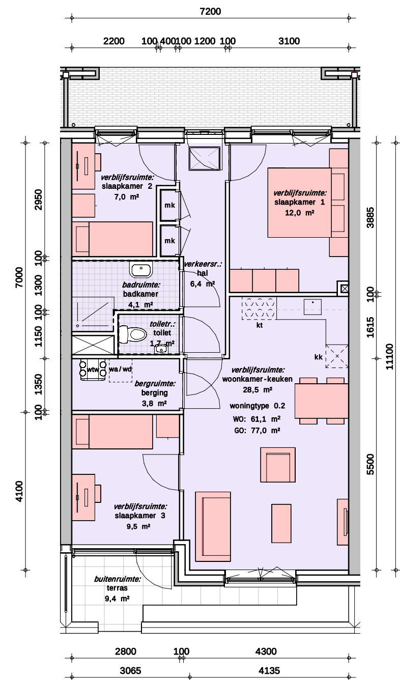
type 0.2b vrije hoogte 3260mm
